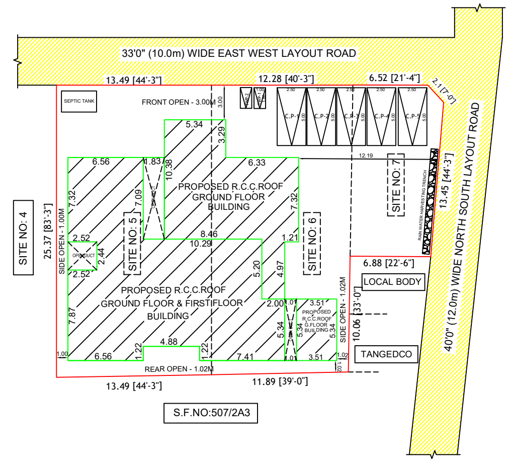
SITE PLAN : 1:200
