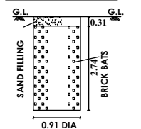
LONGITUDINAL SECTION
