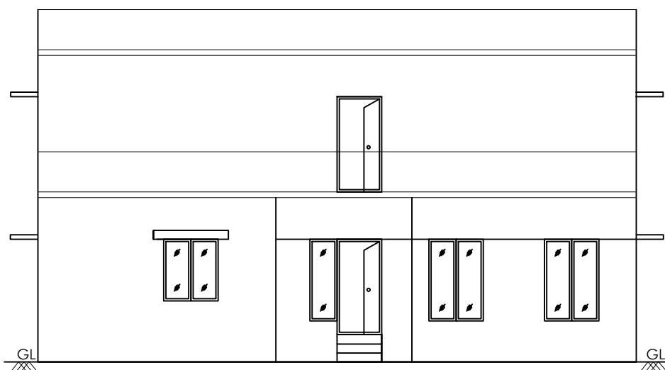
ELEVATION
