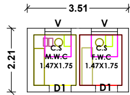
TOILET PLAN
