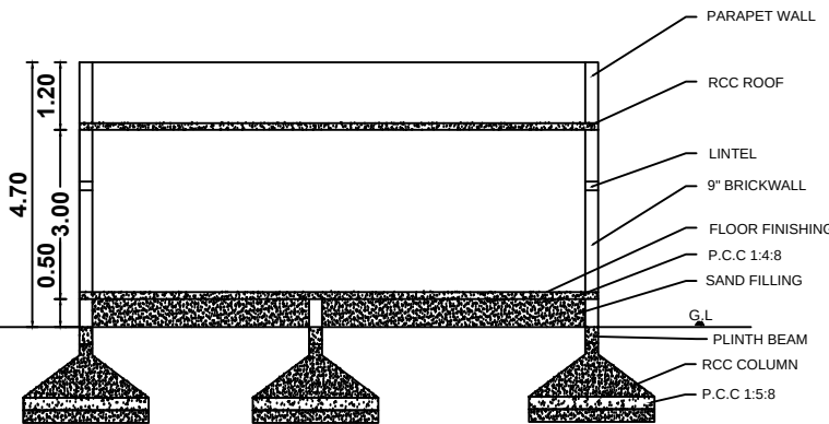
SECTION 'AB'
