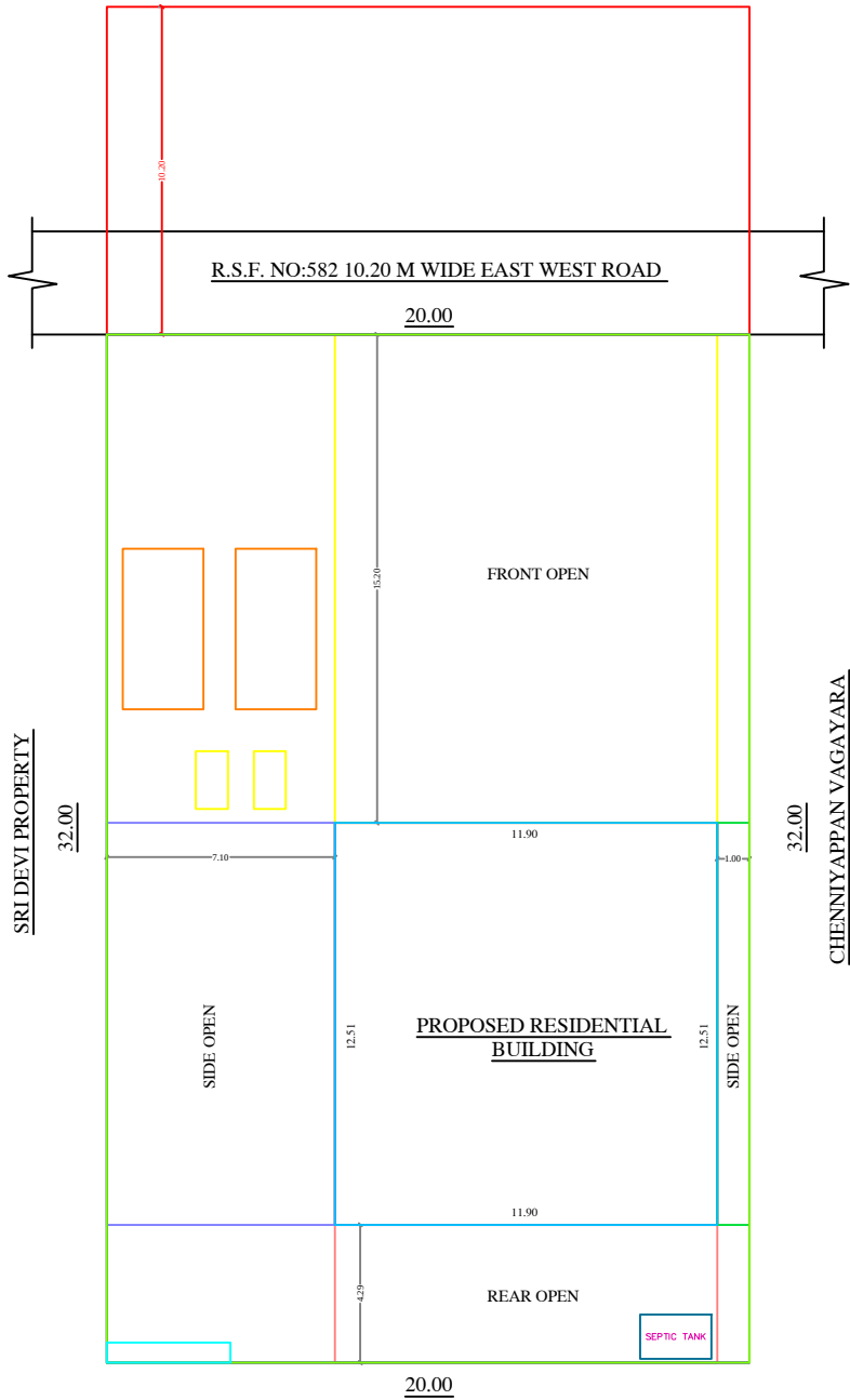
SITE PLAN 1:100
