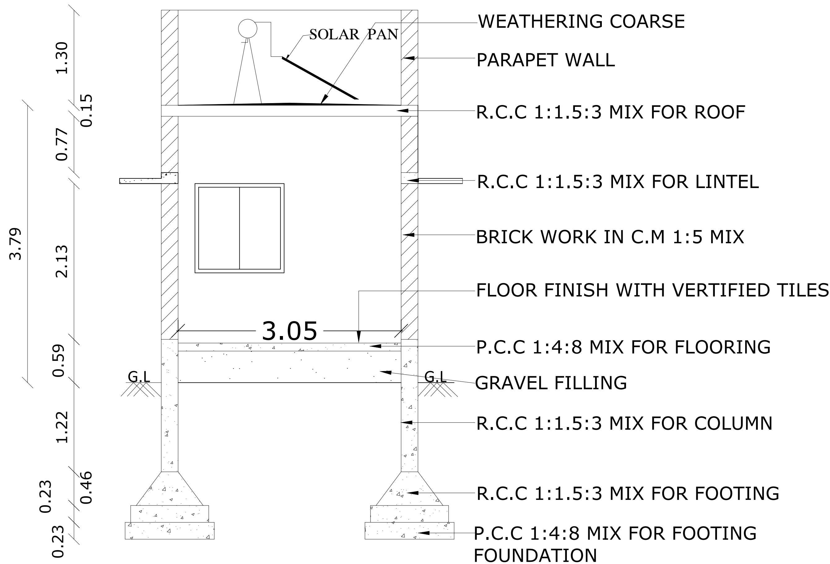
SECTION A-A'
