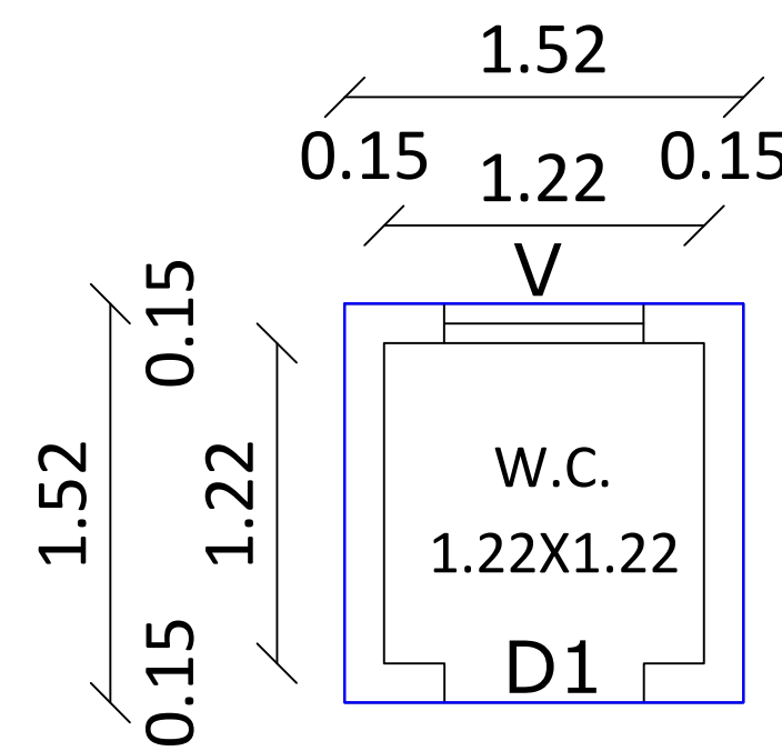
TOILET PLAN
