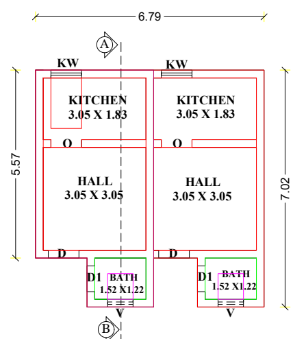
PLAN SCALE : 1:100
