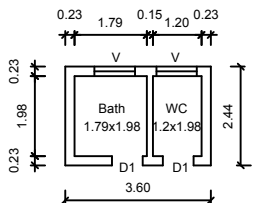
TOILET PLAN
