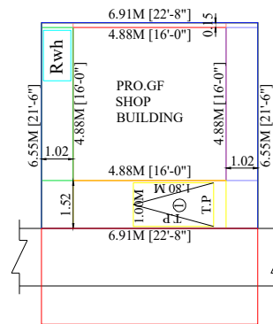
SITE PLAN (NTS)
