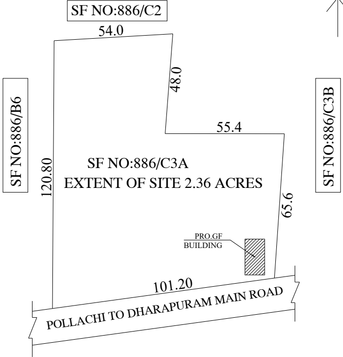
SITE PLAN (NTS)
