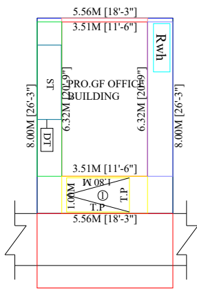
SITE PLAN (NTS)
