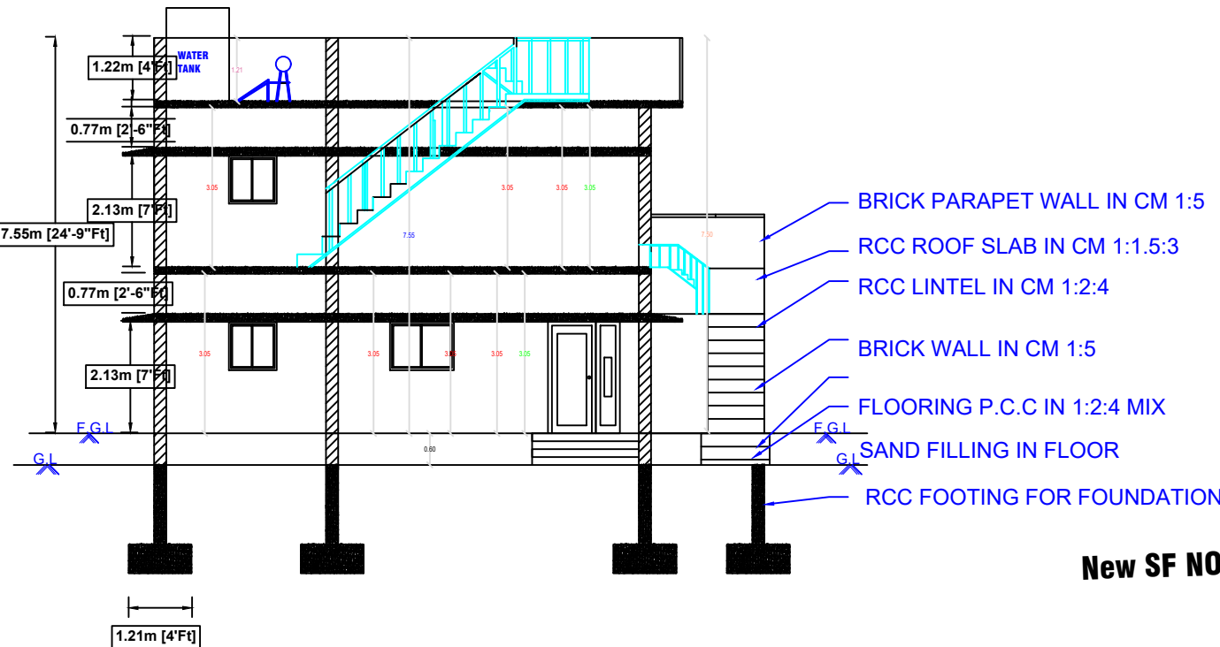
SECTION A-AA
