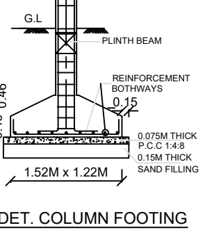
DET. COLUMN FOOTING
