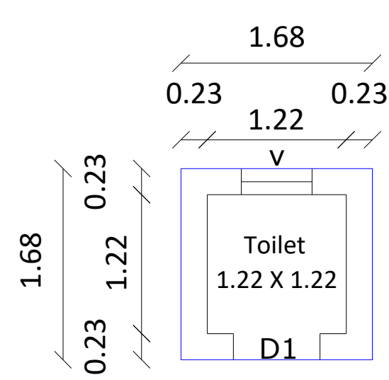
OUTER TOILET
