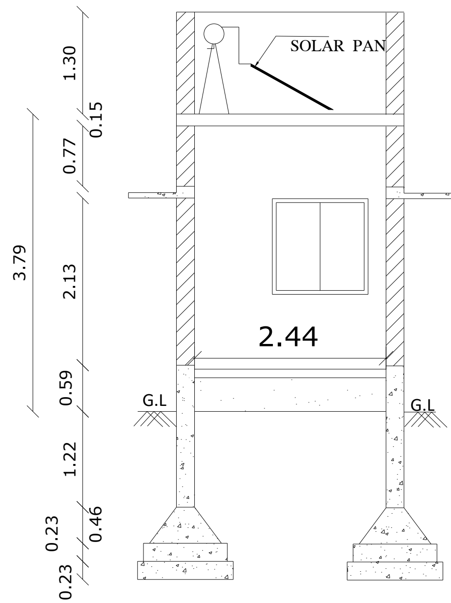
SECTION A-A'
