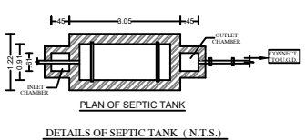
DETAILS OF SEPTIC TANK (N.T.S.)
