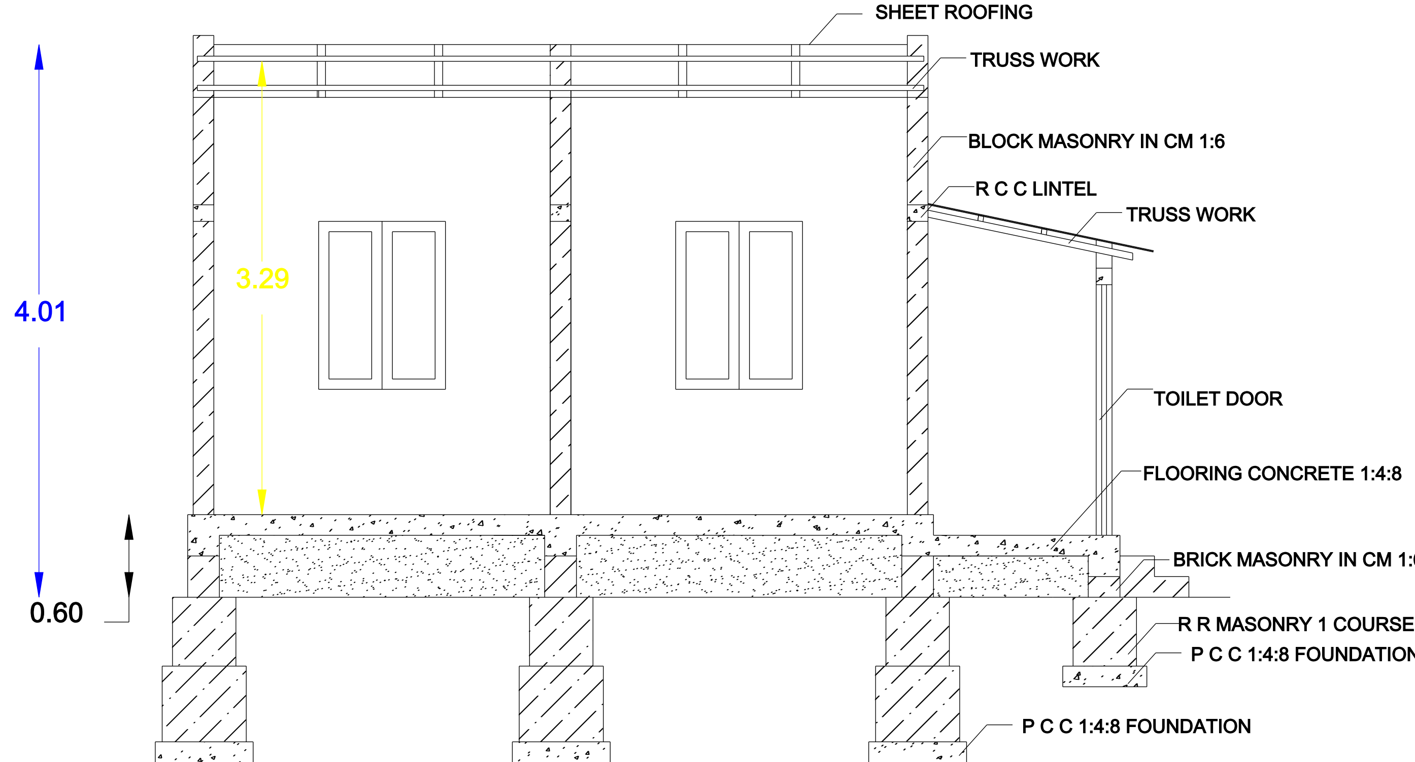
SECTION - AB
