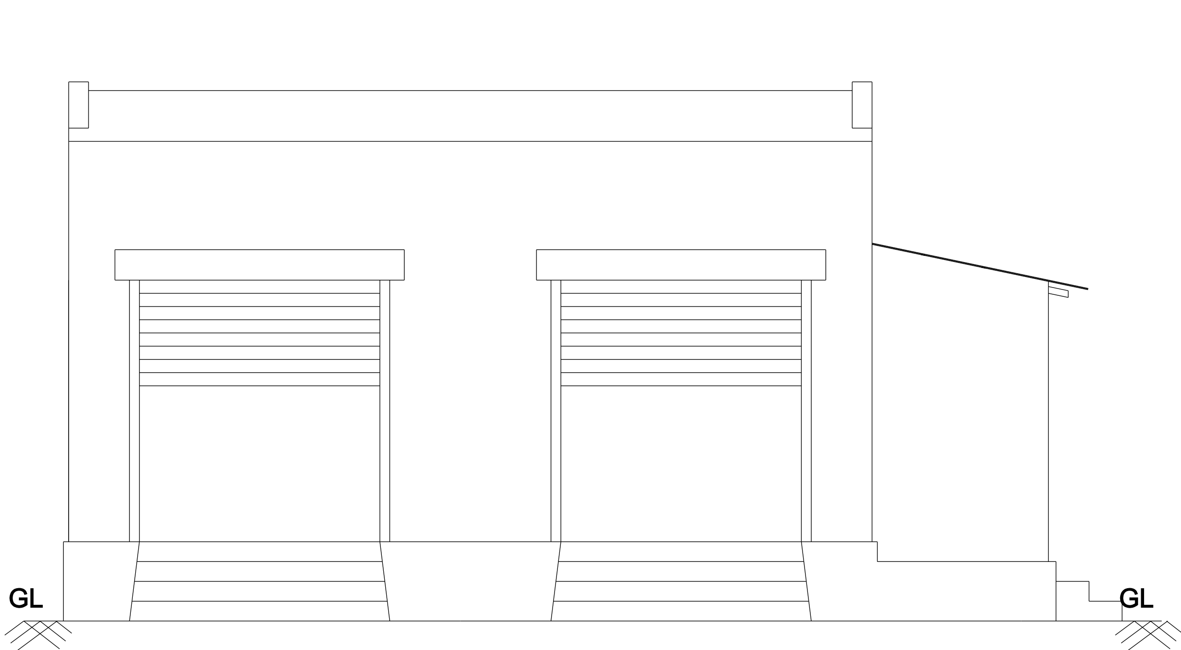
ELEVATION
