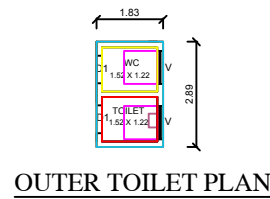
OUTER TOILET PLAN
