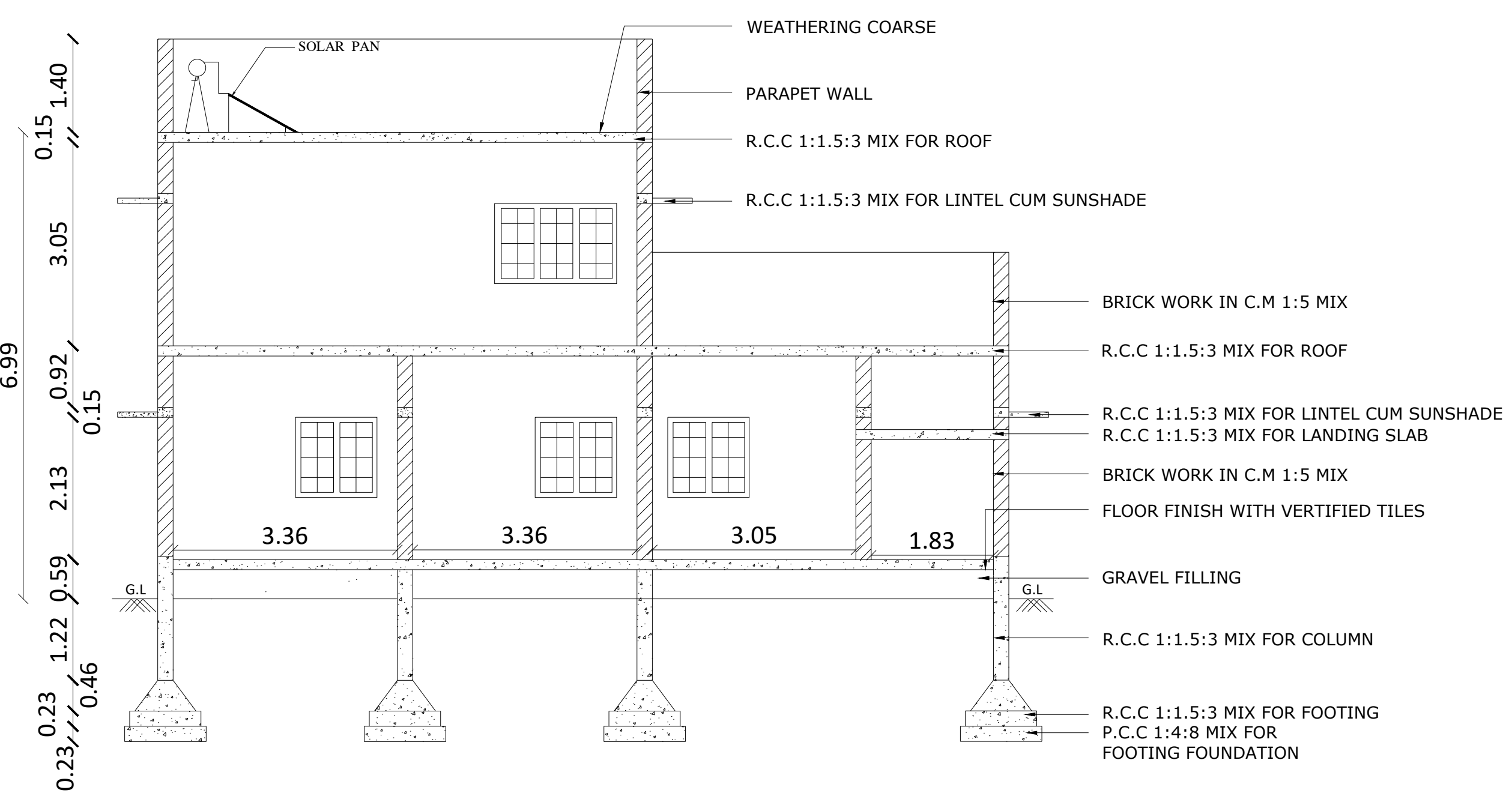
SECTION A-A'
