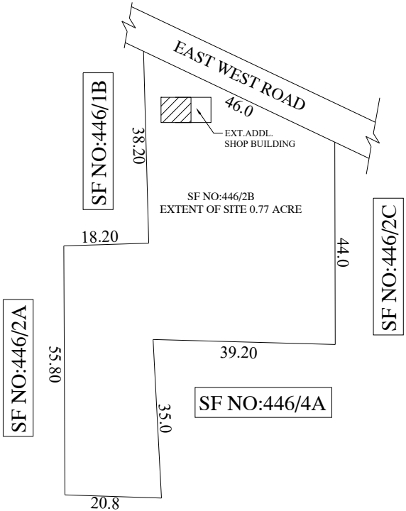
SITE PLAN (NTS)
