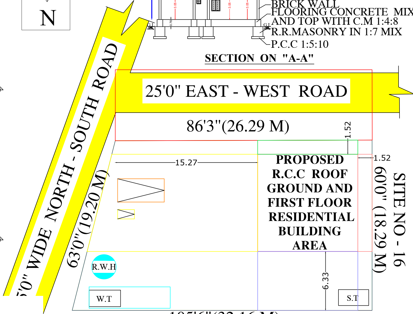
SITE NO - 2 SITE PLAN
