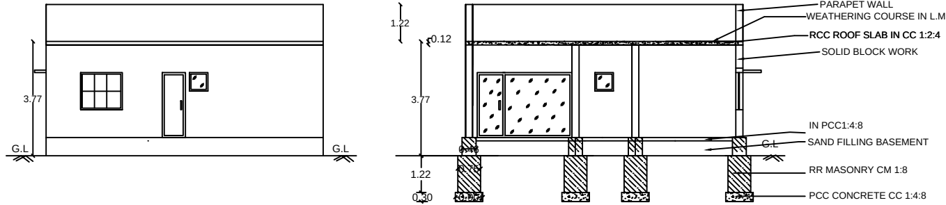
ELEVATION
