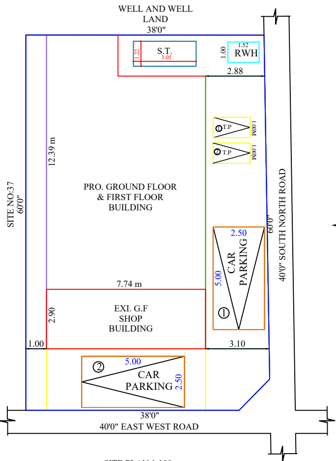
SITE PLAN 1:100
