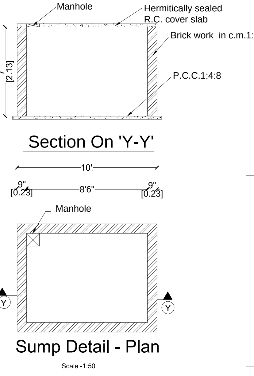
Sump Detail - Plan Scale: 1:50
