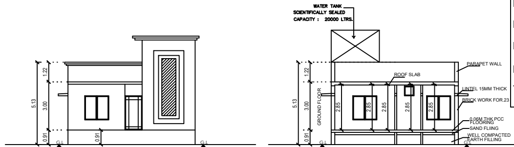
ELEVATION
