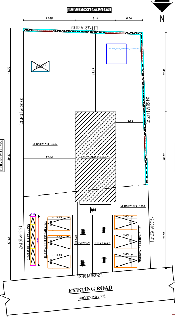
SITE PLAN ( 1 : 200 )
