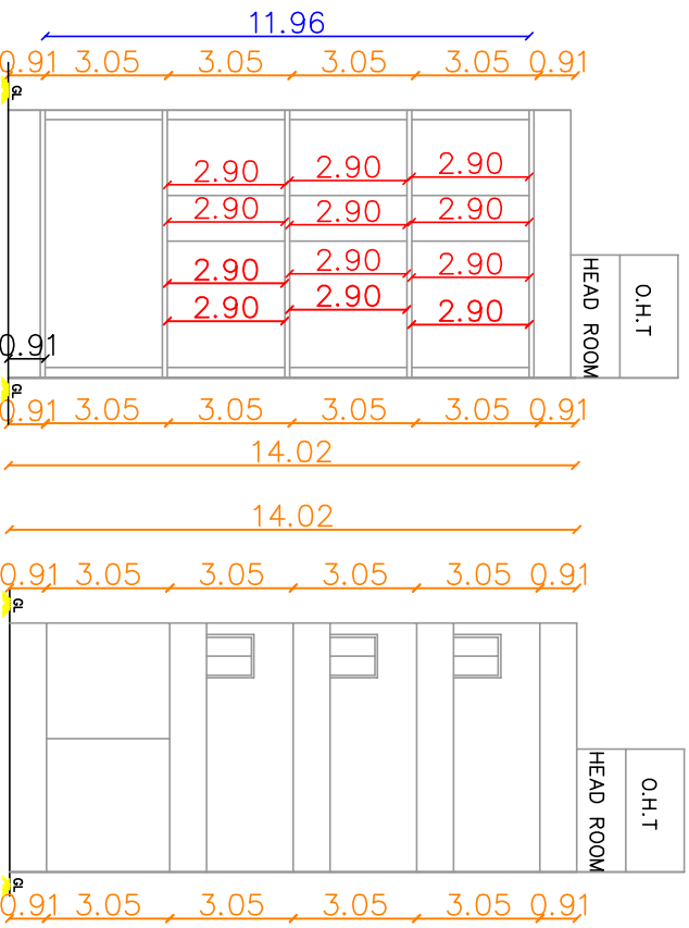
ELEVATION ELEVATION
