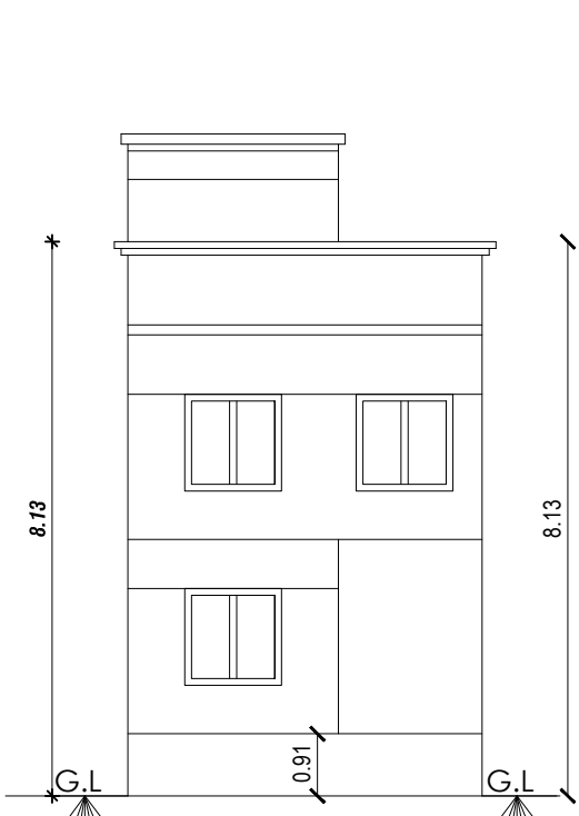
ELEVATION
