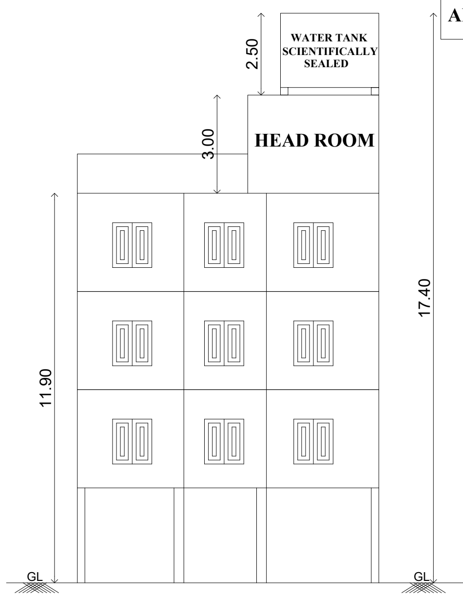
ELEVATION
