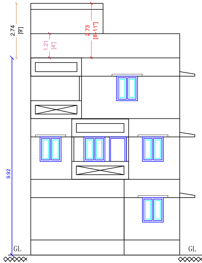
ELEVATION
