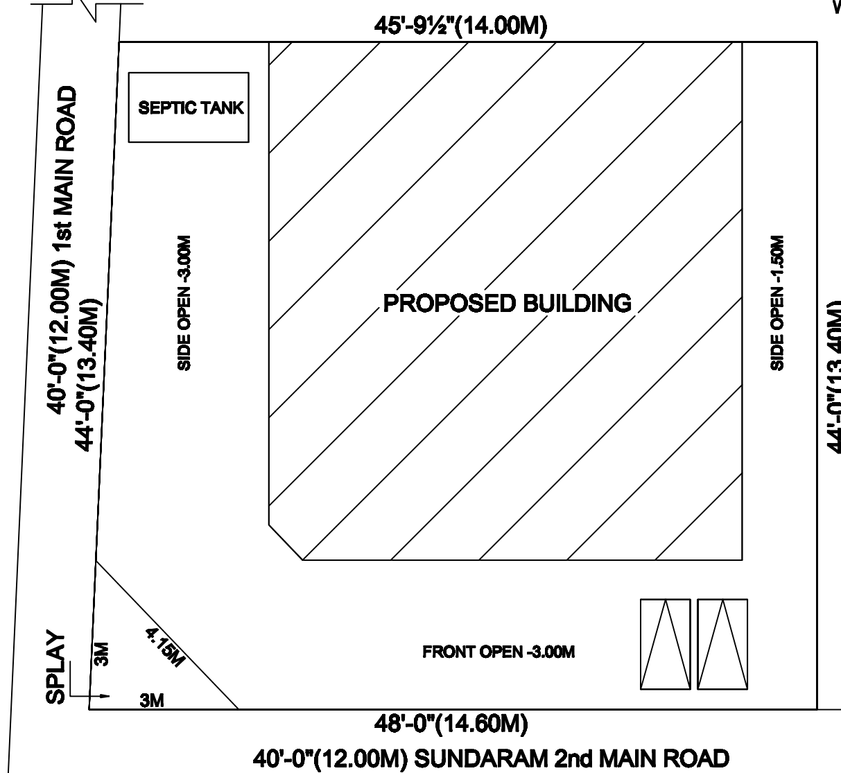
SITE / PLAN
