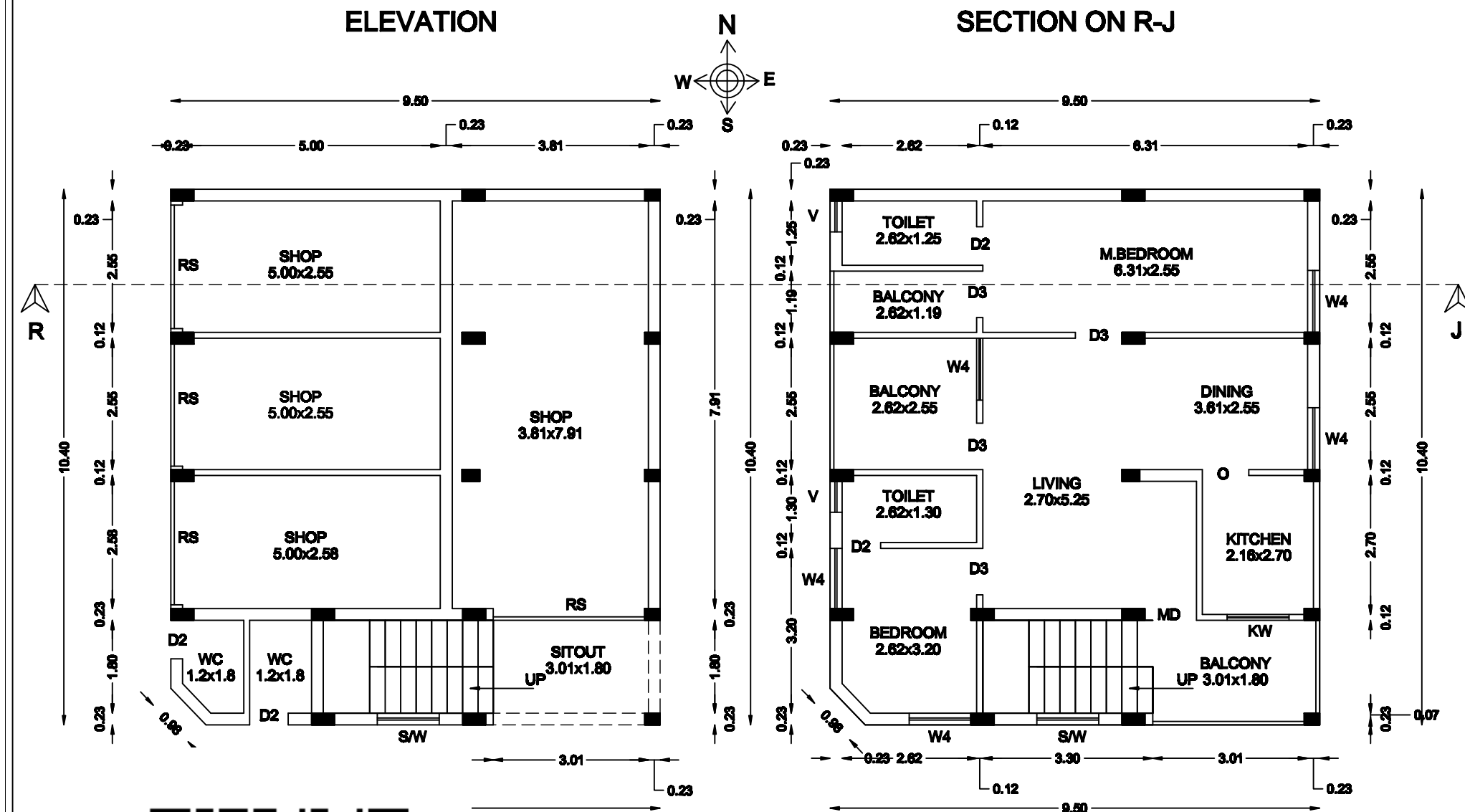
DR PLAN
