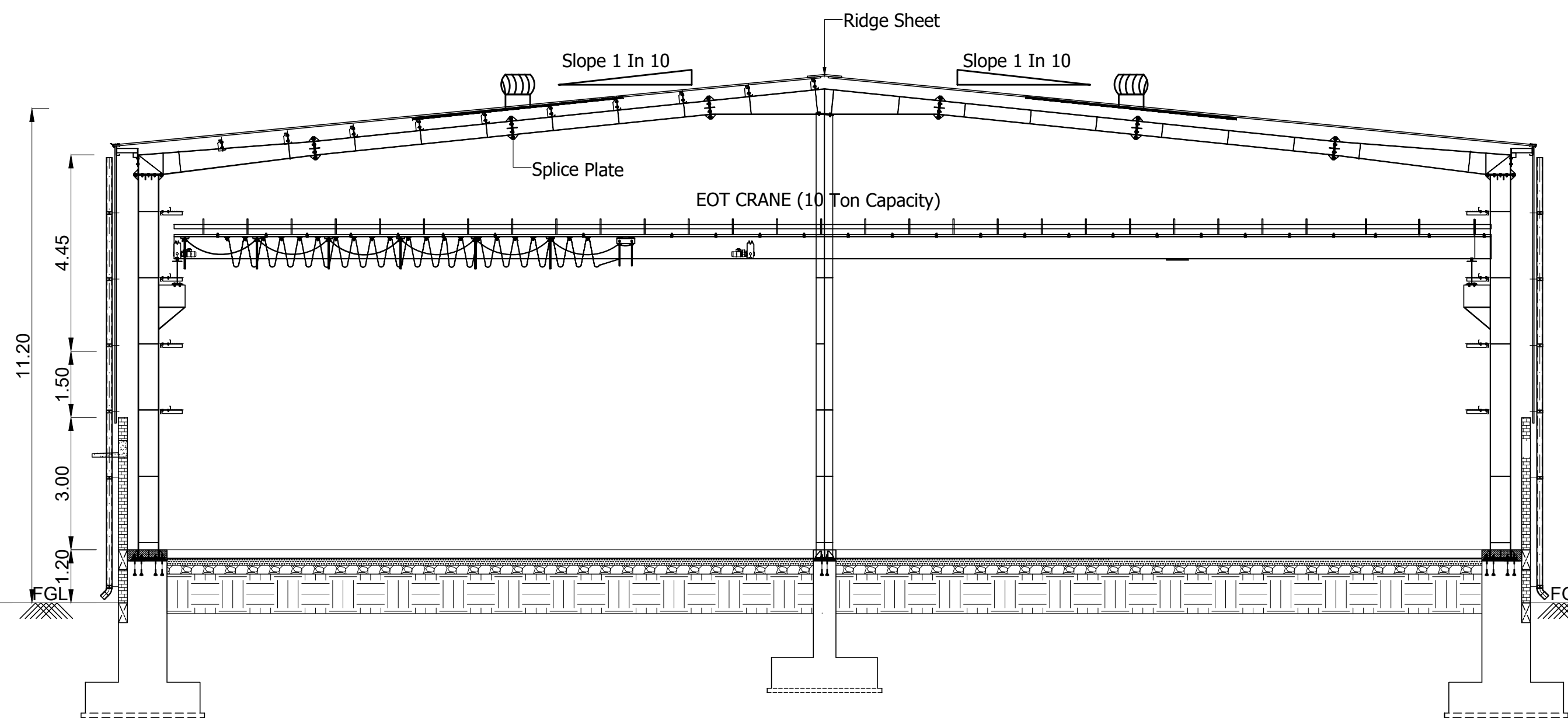
SECTION D-D
