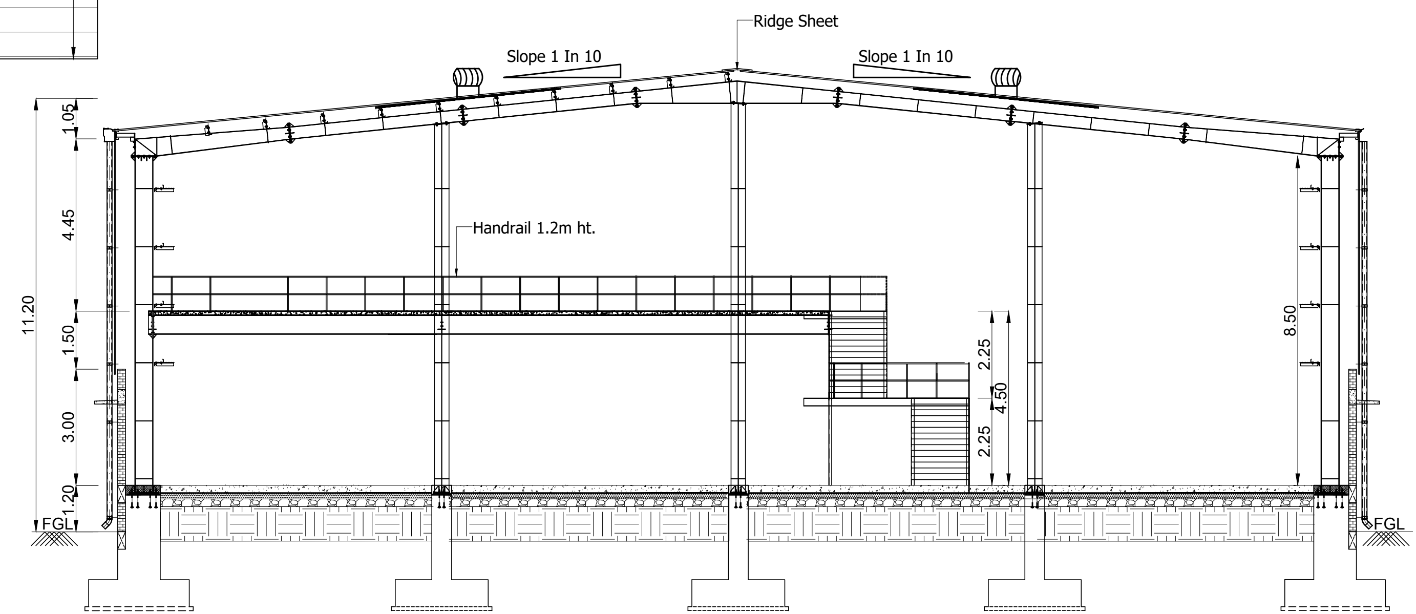
SECTION A-A
