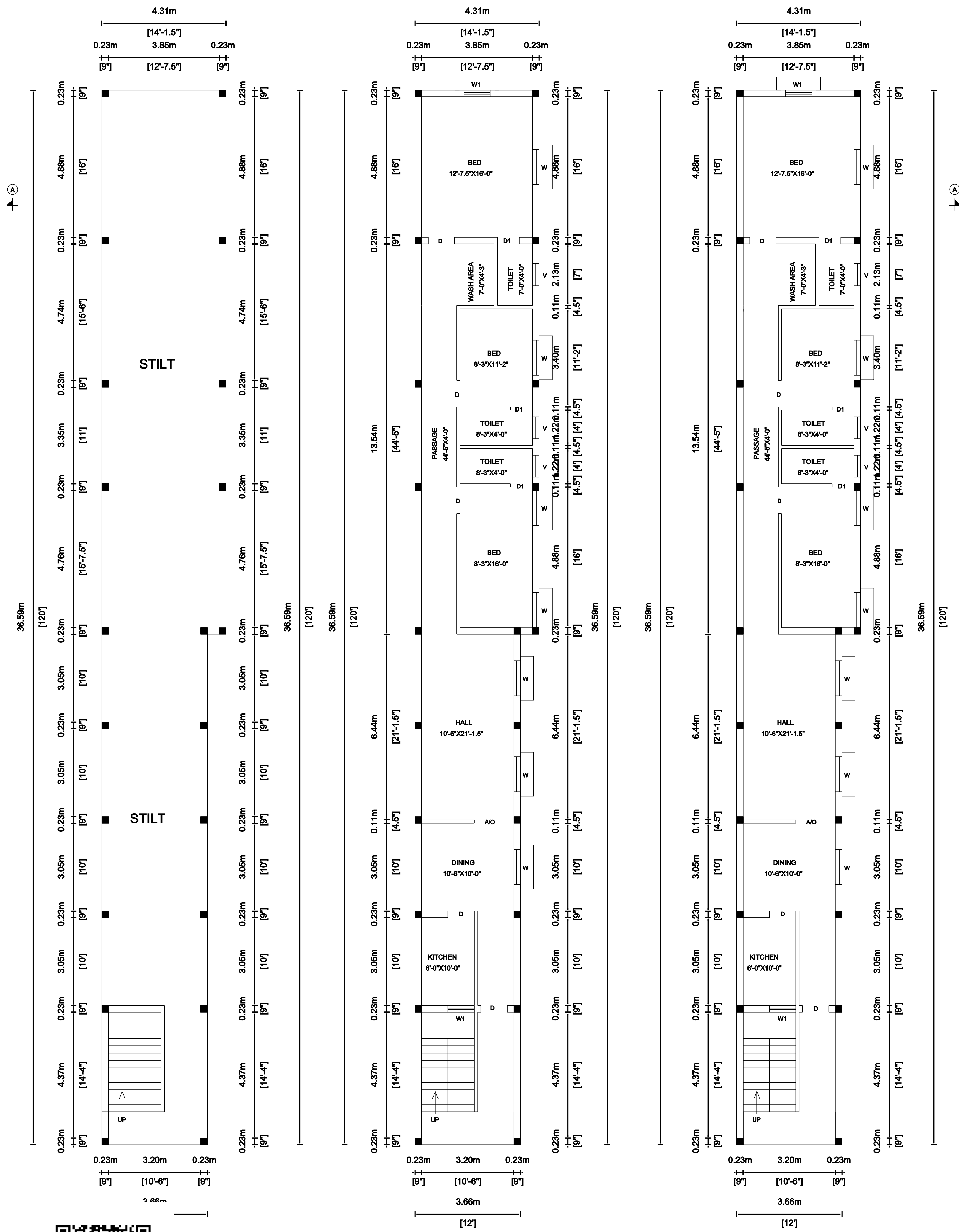
STILT) PLAN
