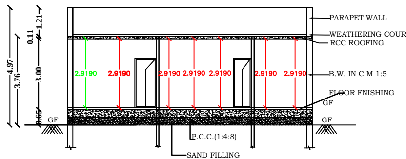
SECTION A-B
