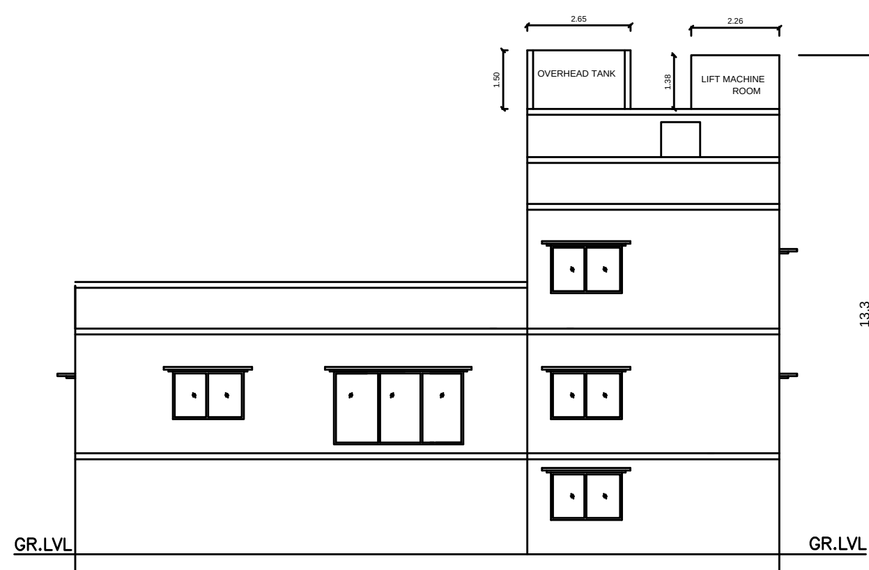
ELEVATION
