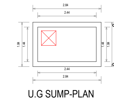
U.G SUMP-PLAN
