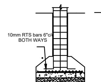
FOUNDATION SCALE: 1:50 (1" = 4'0")
