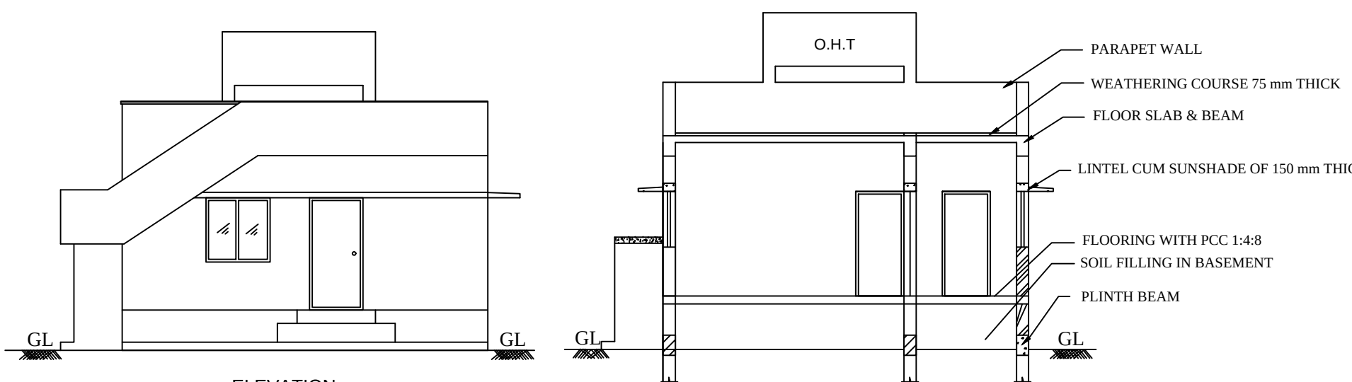
SECTION A-A
