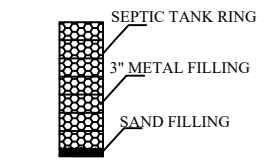
R.W.H DETAILS
