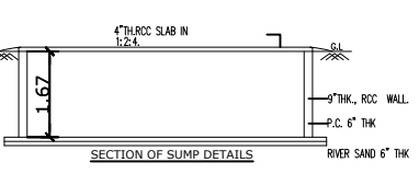
R.W.H DETAILS
