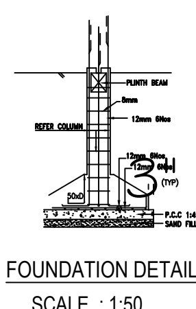
SCALE : 1:50.
