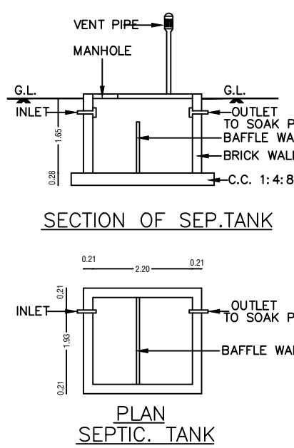
SCALE : 1:50.
