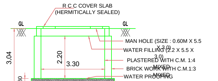
SECTION ON DD
