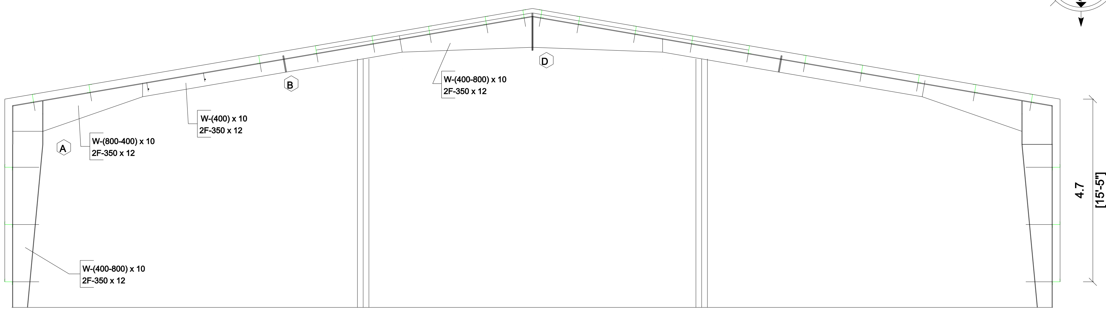
ELEVATION
