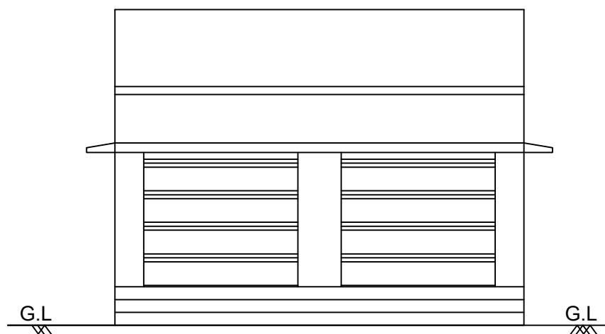
ELEVATION
