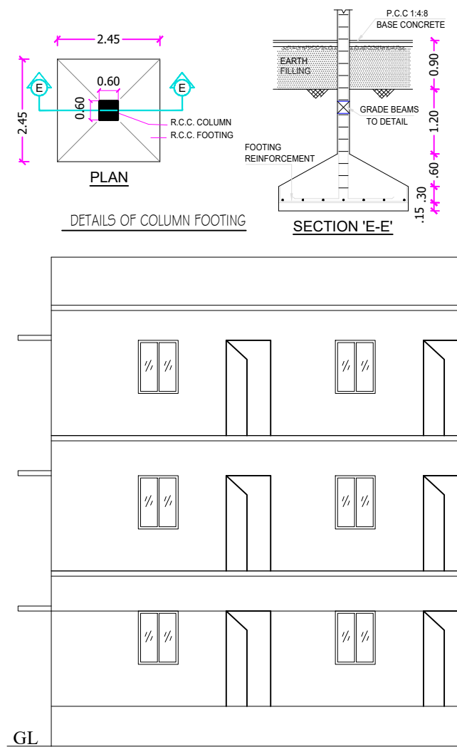
ELEVATION
