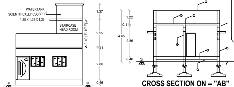
ELEVATION
