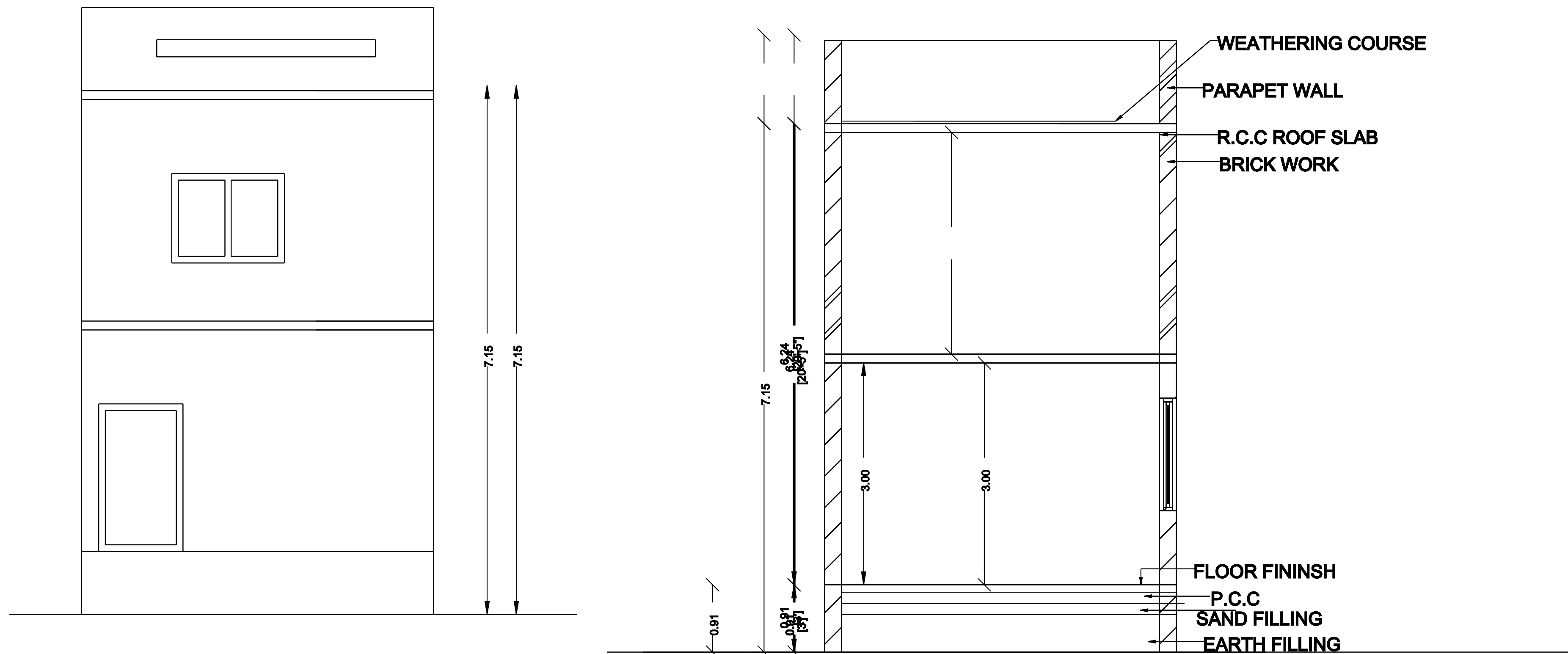
ELEVATION
