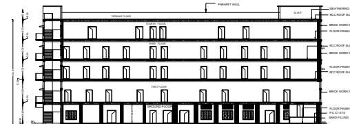
SECTION -JS
