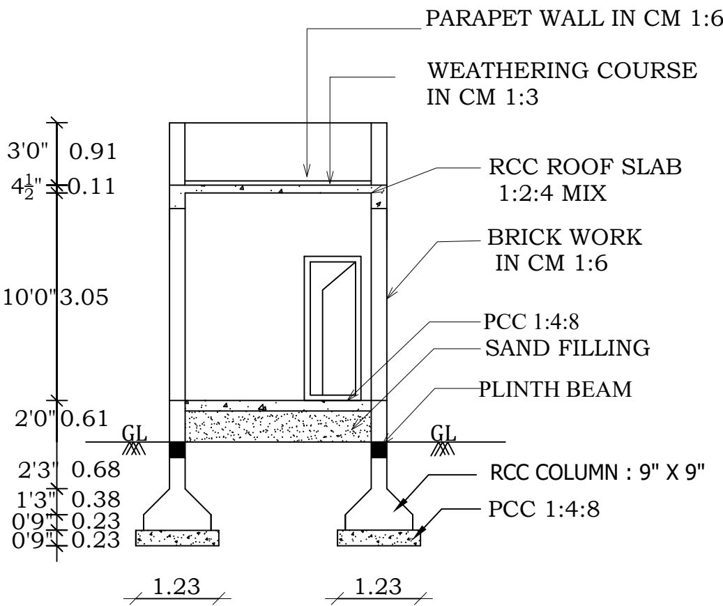
SECTION - AB
