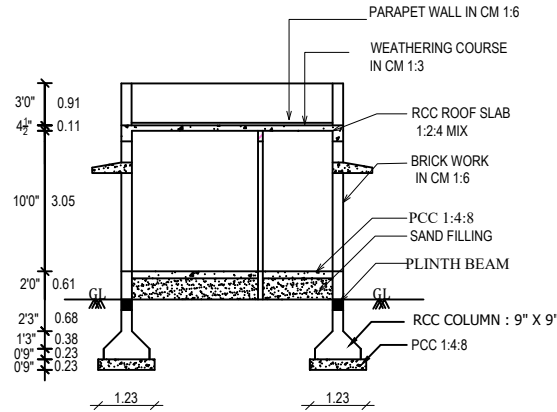
SECTION - AB
