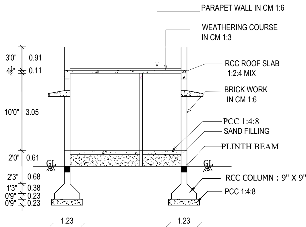
SECTION - AB
