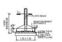
TYP. DET. COLUMN FOOTING
